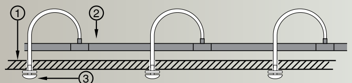
1: Tak, 2: Aspirasjonsrør, 3: Sniffer
