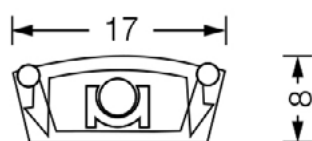
Innfelling/påvegg
